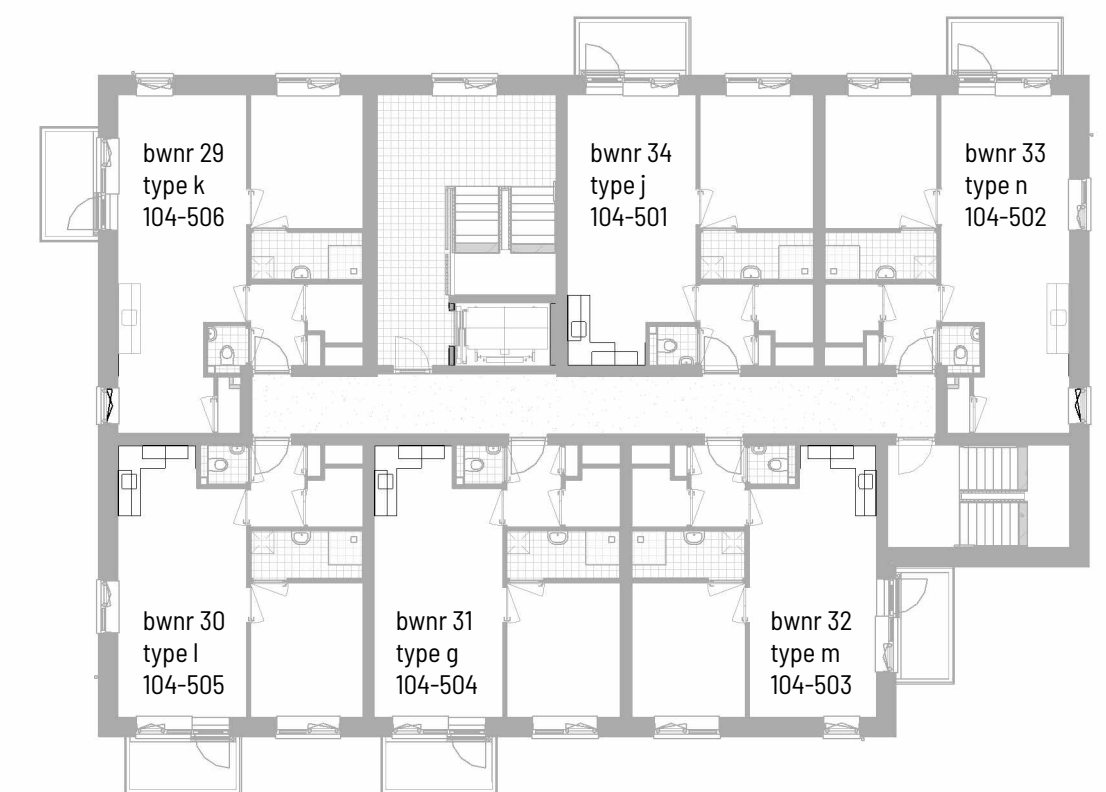
vijfde verdieping 1: 200
