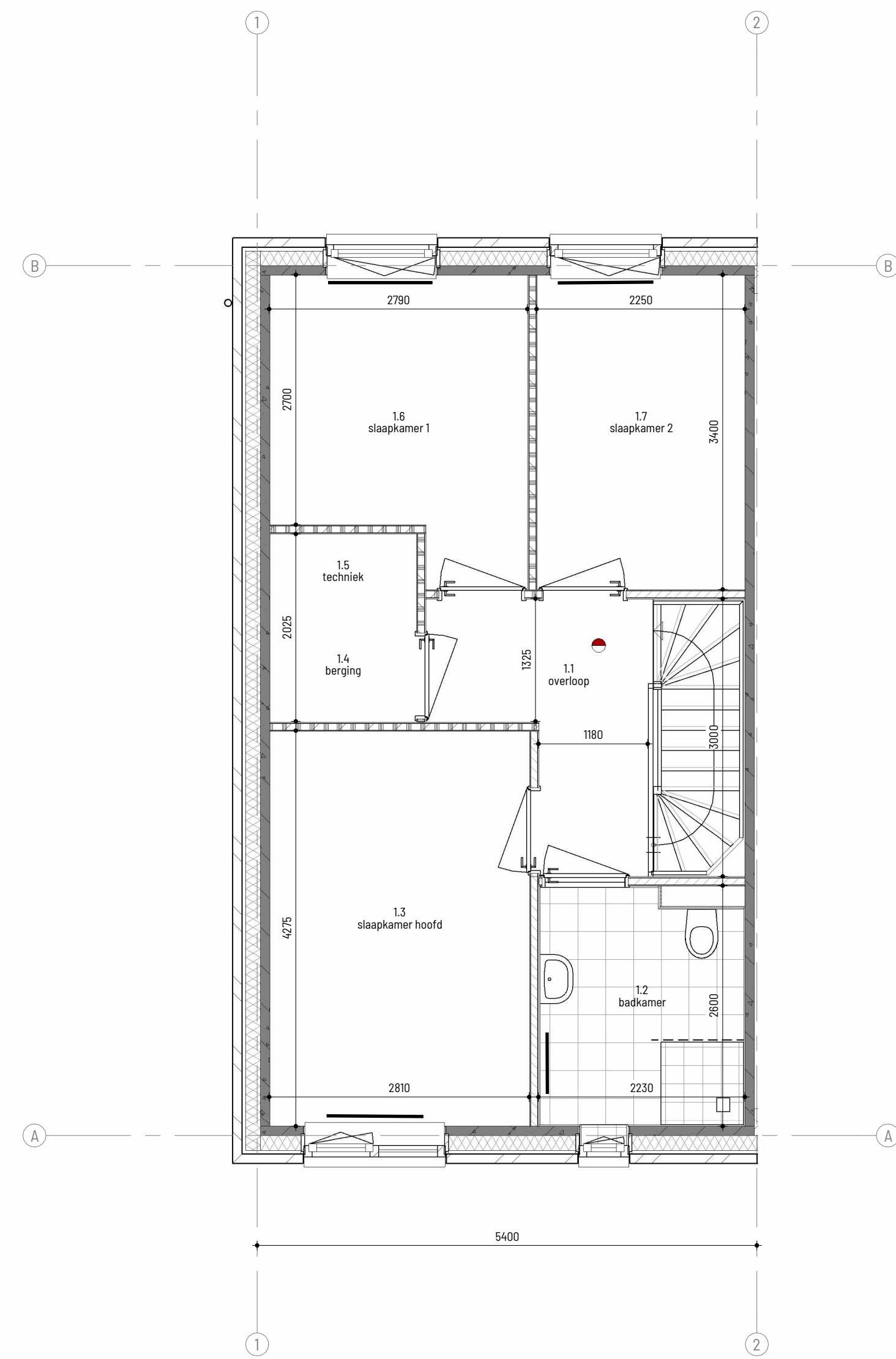
eerste verdieping
