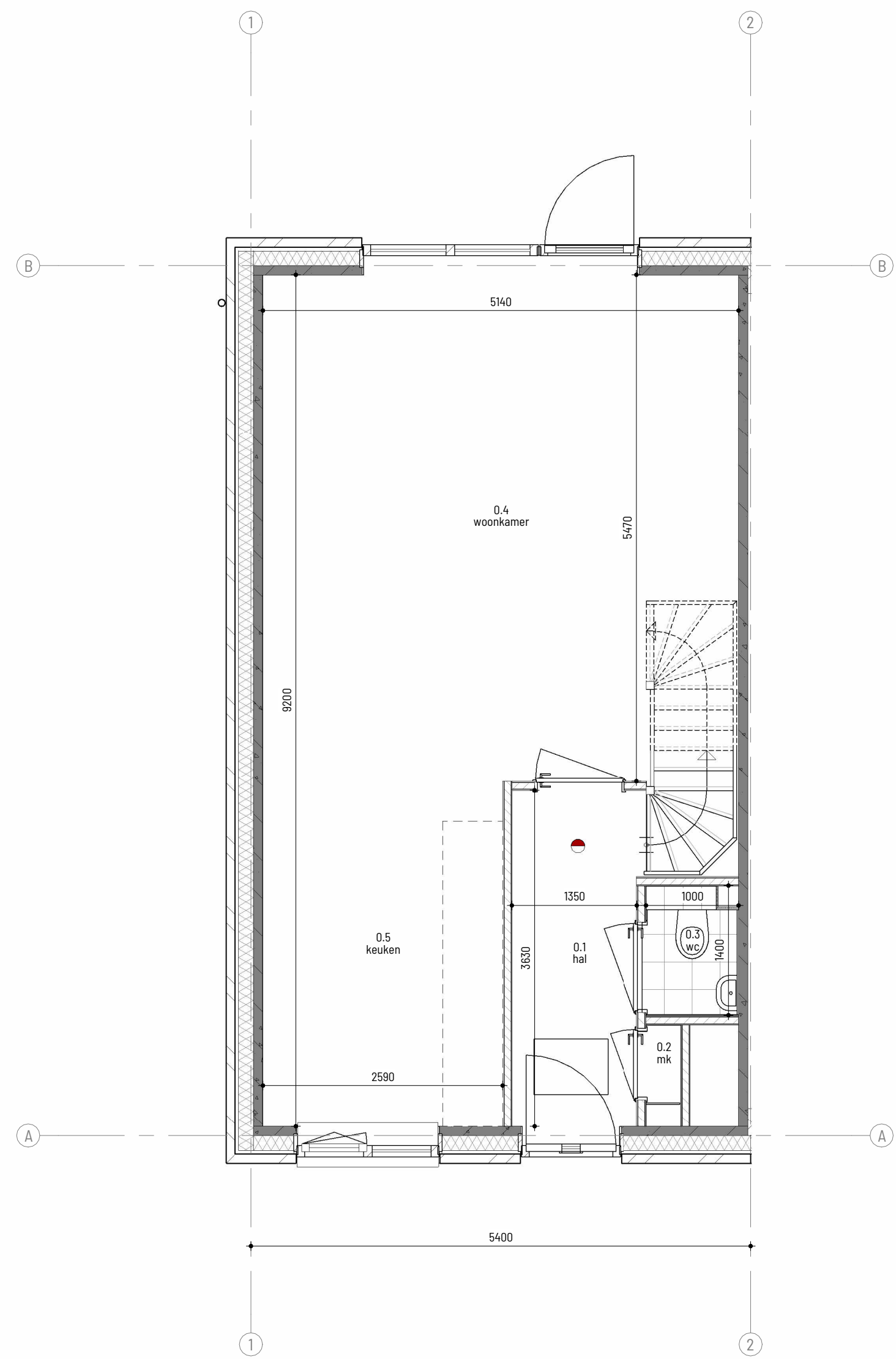
begane grond
