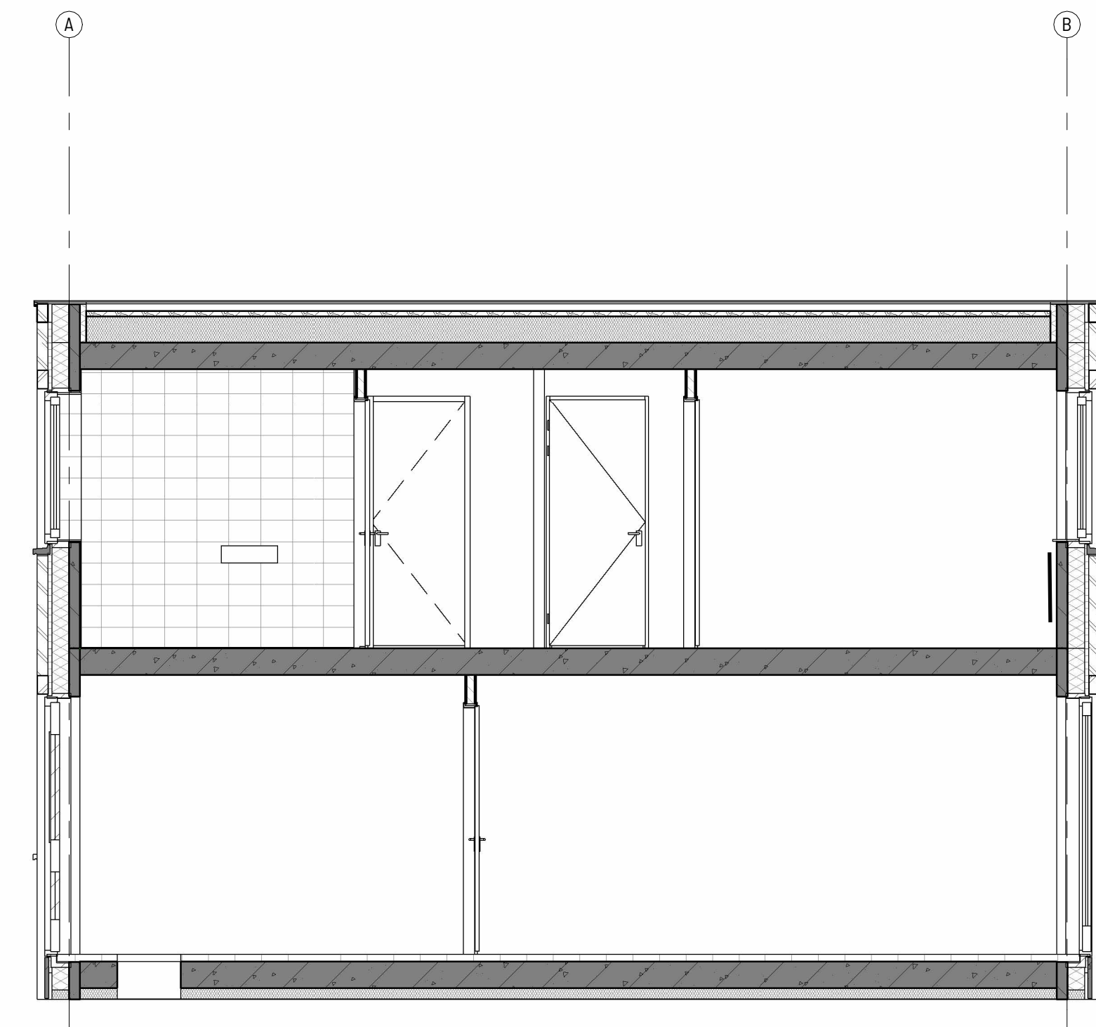
doorsnede
