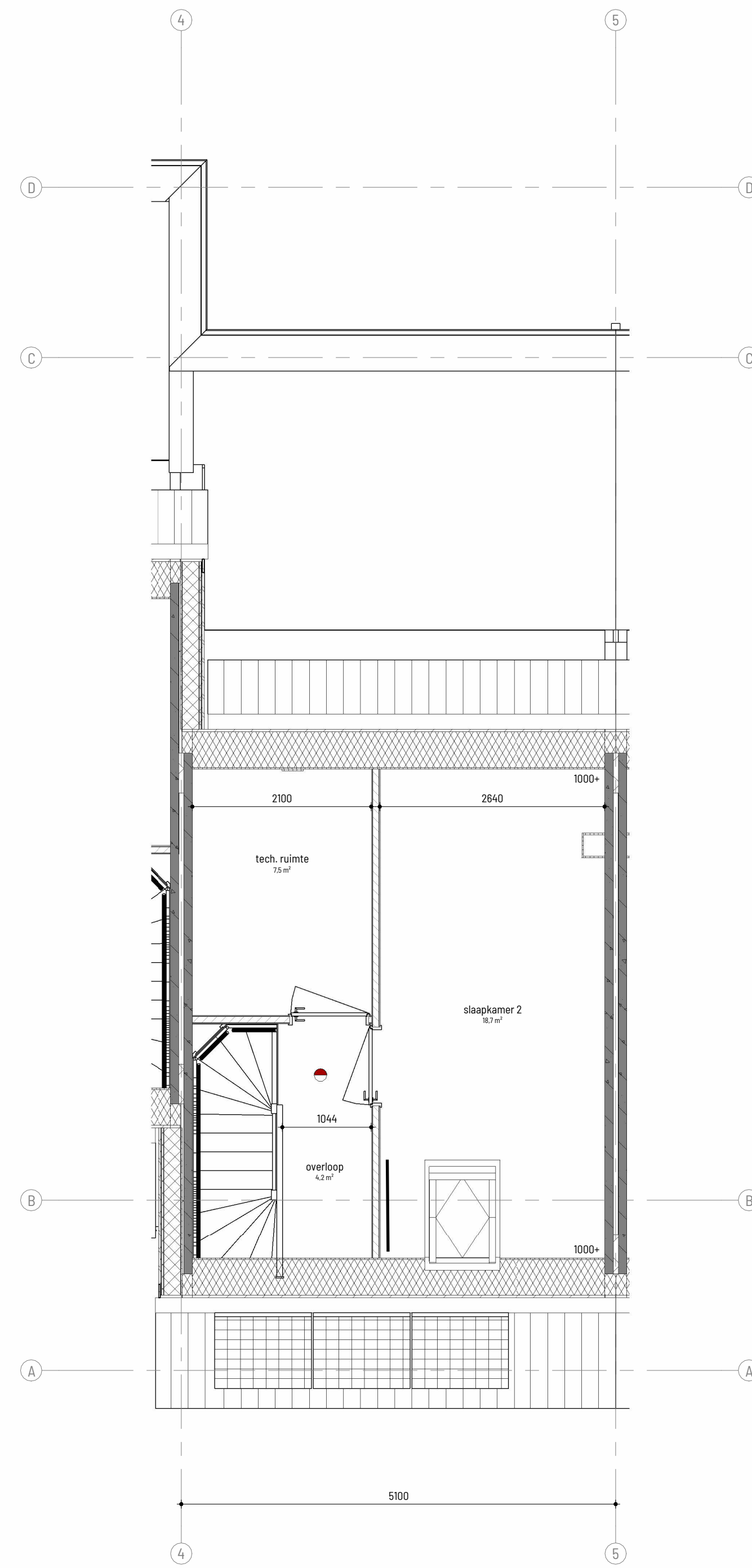
eerste verdieping
