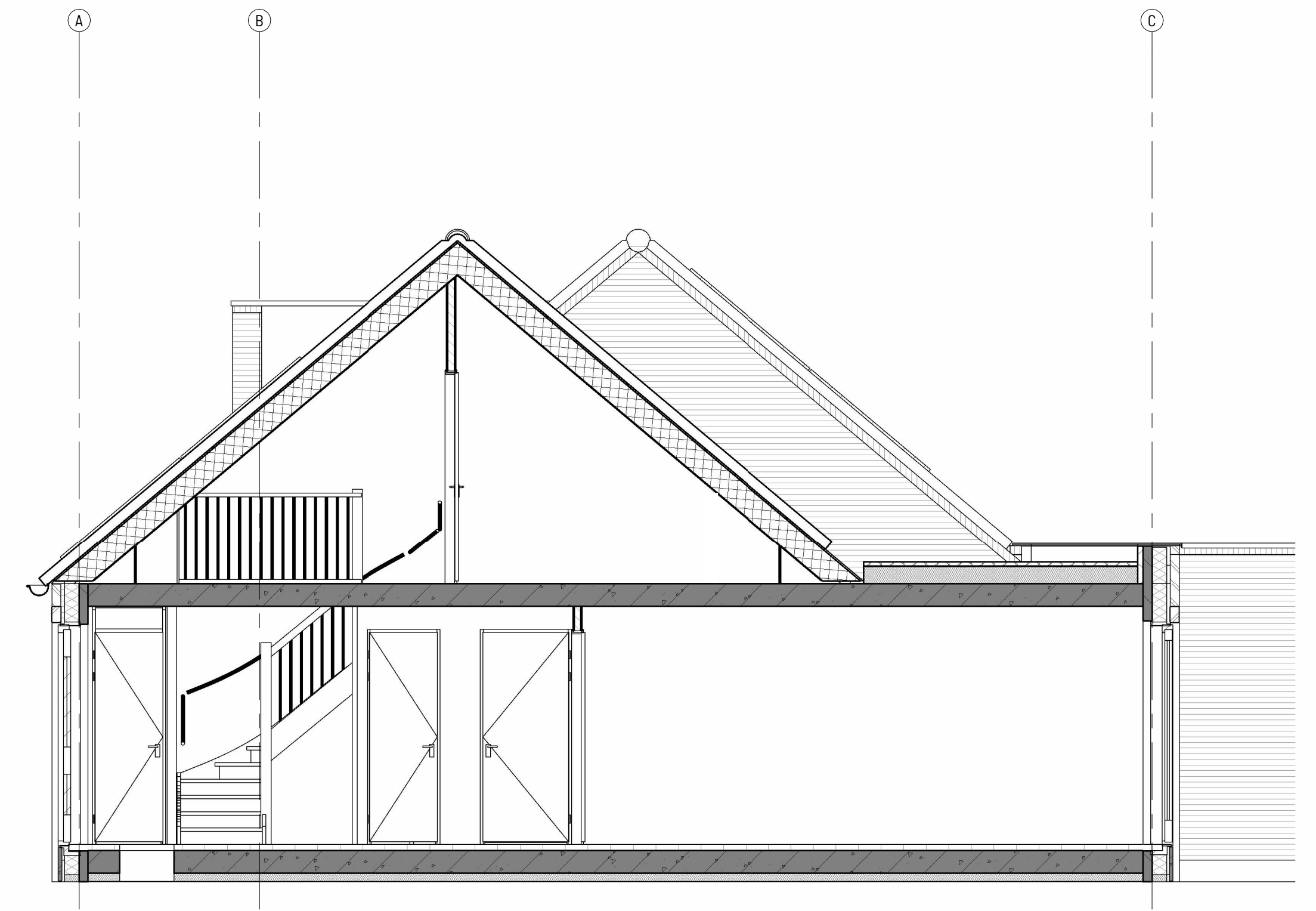
doorsnede
