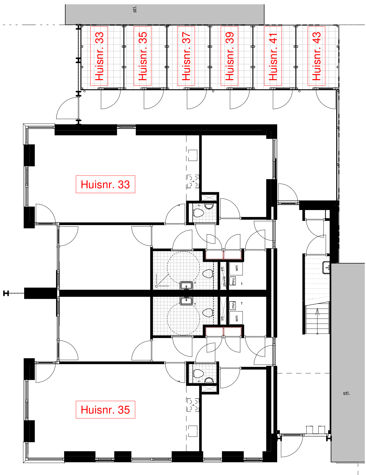
DRIENERWEG begane grond
