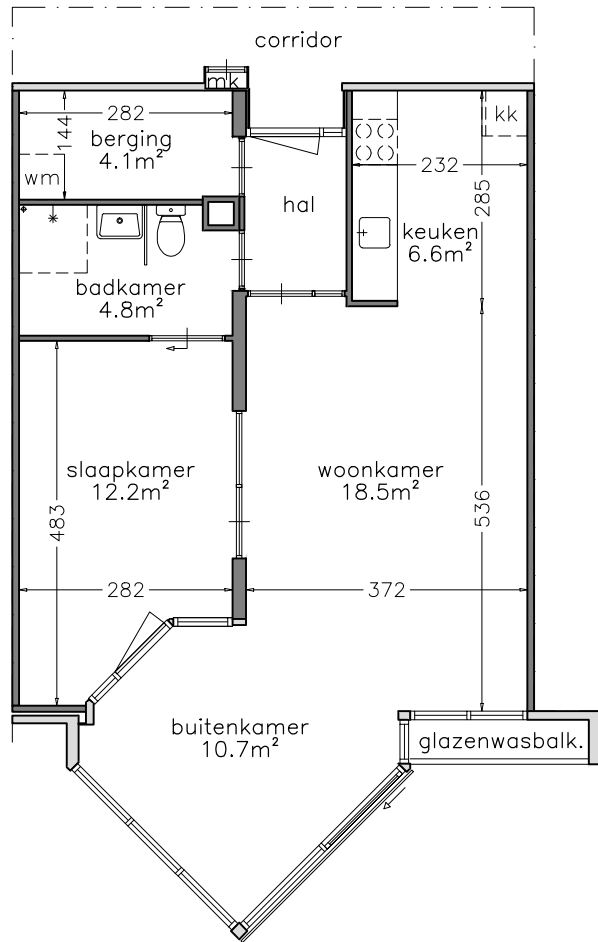
verdieping 6 woningtype A
