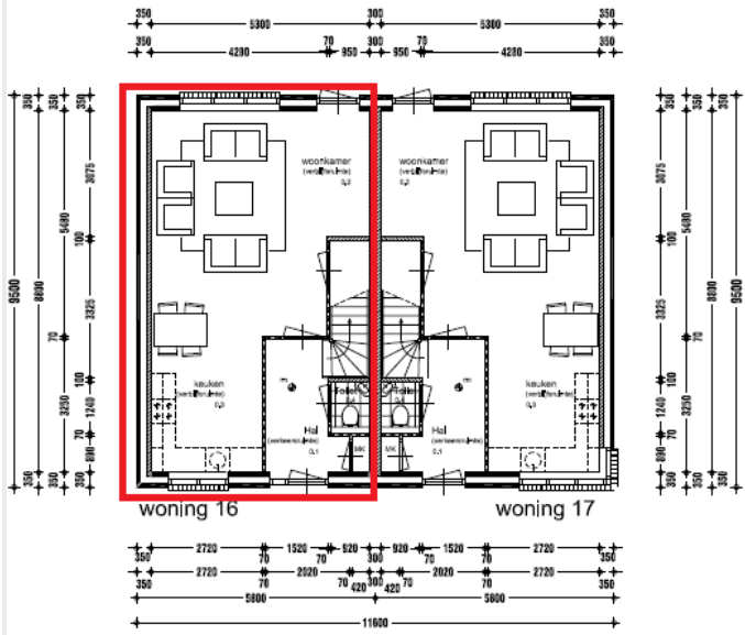
Begane grond
