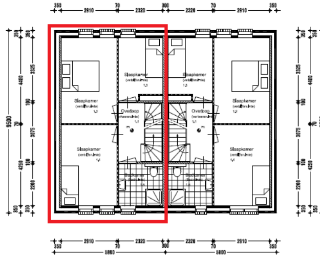
Verdieping
